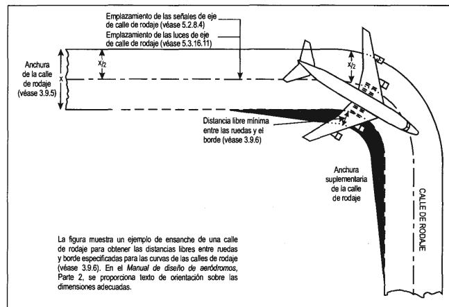
Figura 3 - 2. Curva de calle de rodaje
