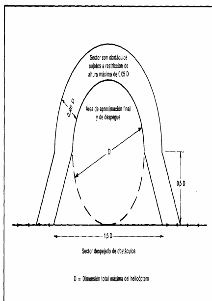
Figura 4-12H. Superficies limitadoras de obstáculos en los helipuertos no construidos para fines especiales en el costado del buque
