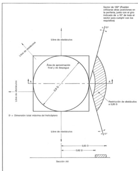
Figura 4-4H. Sectores limitadores de obstáculos en la heliplataforma Helicópteros de rotor principal en tándem - Operaciones omnidireccionales
