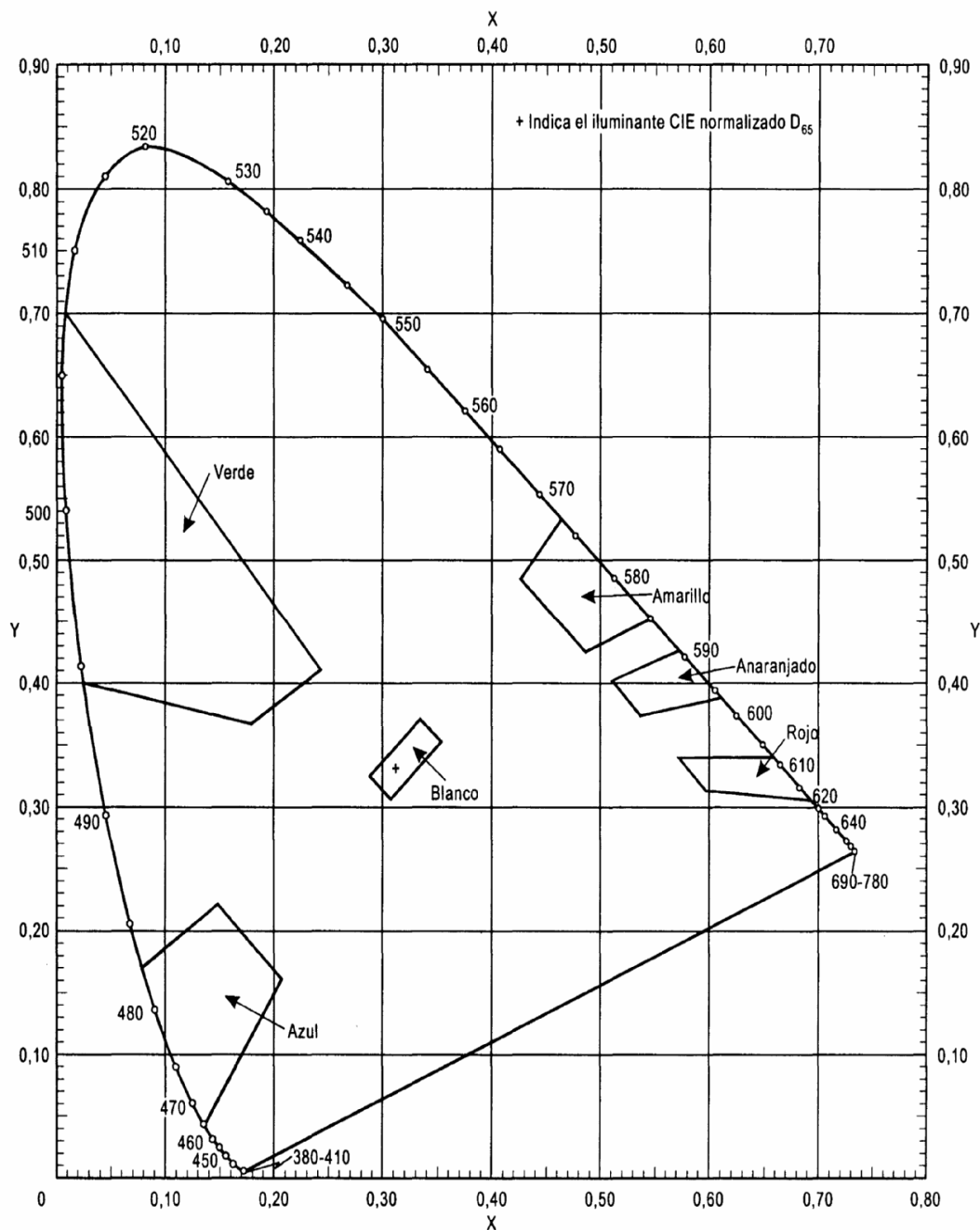
Figura A1 - 3. Colores de los materiales retrorrefletantes para las señales, letreros y tableros
