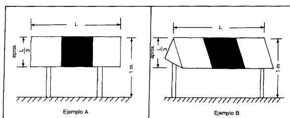
Figura 5-7H. Baliza de ruta de desplazamiento aéreo
