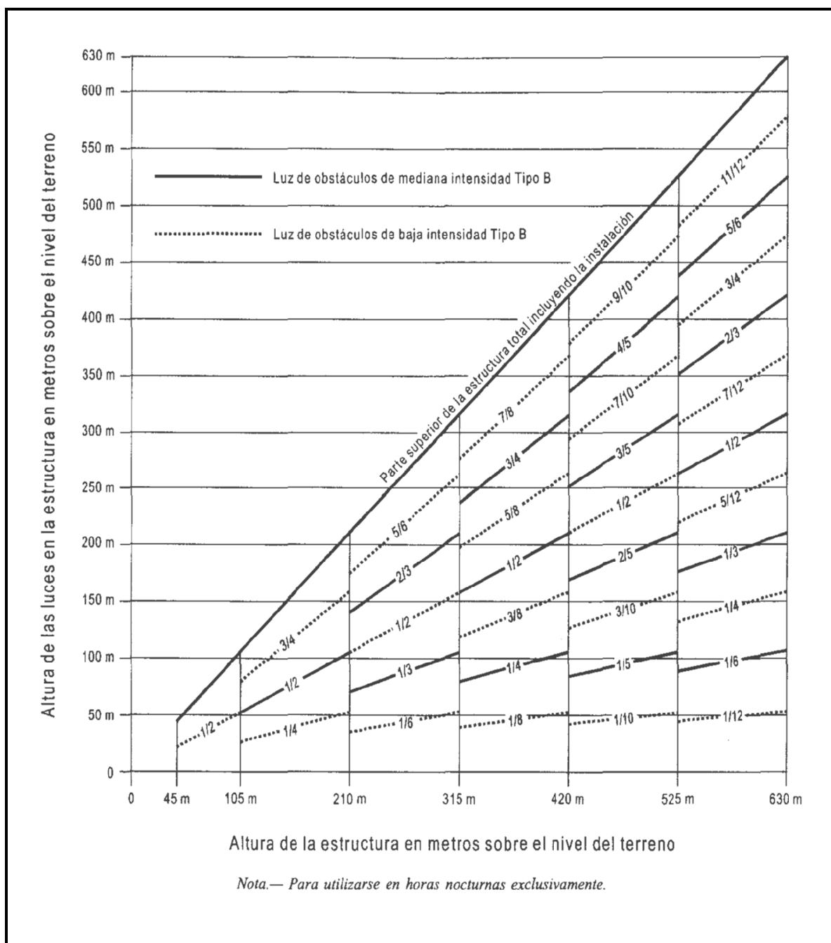
Figura A6 - 2. Sistema de iluminación de obstáculos con luces rojas de destello de mediana intensidad Tipo B
