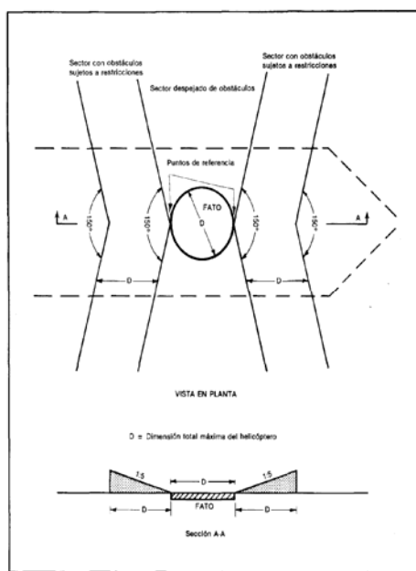
Figura 4-11H. Superficies limitadoras de obstáculos en los helipuertos no construidos para fines especiales en el centro del buque
