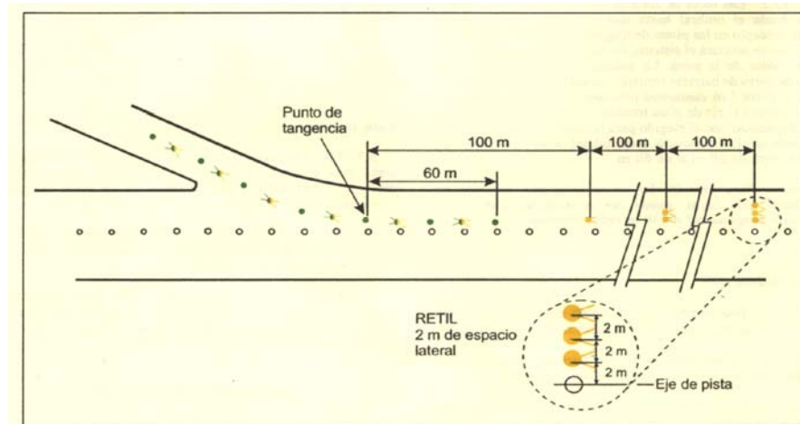
Figura 5-23. Luces indicadoras de la calle de salida rápida
