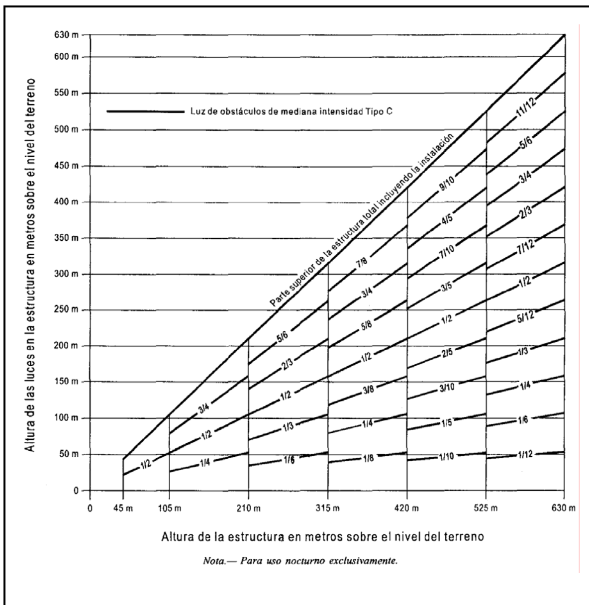
Figura A6 - 3. Sistema de iluminación de obstáculos con luces rojas fijas de mediana intensidad Tipo C
